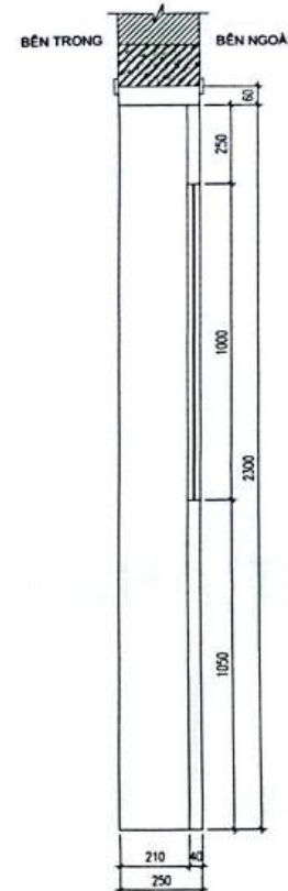
MẶT CẮT DỌC
