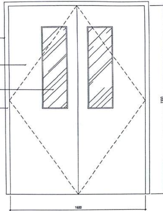
MẶT ĐỨNG
