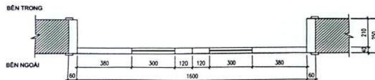
MẶT CẮT NGANG
